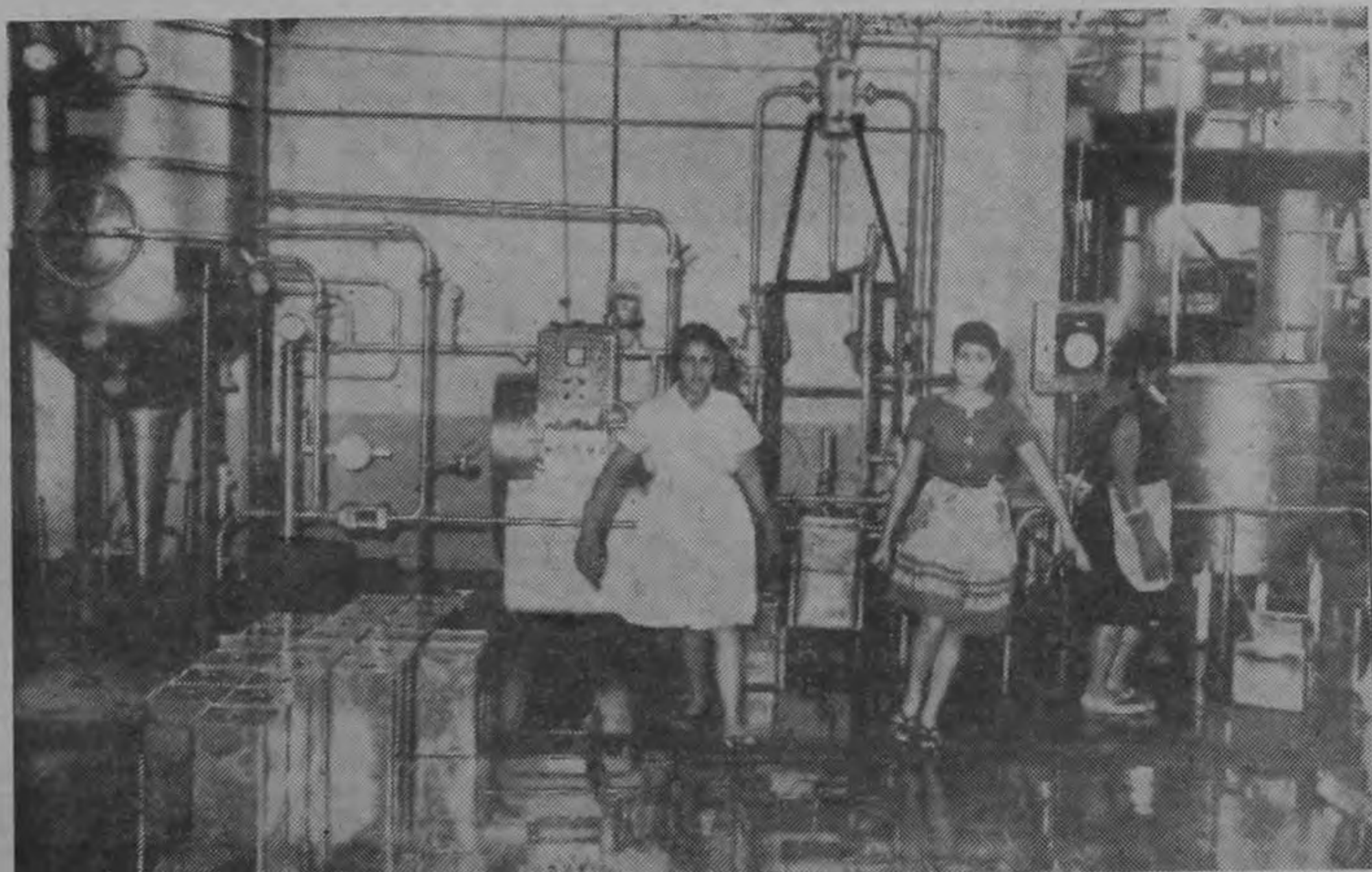
A la izquierda, "desintegrador al vacío", que produce una homogeneización altamente perfeccionada junto con el rapid-sonic. A la derecha la centrifugadora, que elimina de la pulpa cualquier materia extraña al producto, por pequeña que sea. El Dr. Bertuzzi, un científico, más que un industrial, puso todo su conocimiento en su equipo, que está instalado en todos los continentes y en más de cincuenta países.
